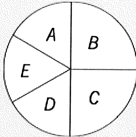
Fig. 3 Pie task
